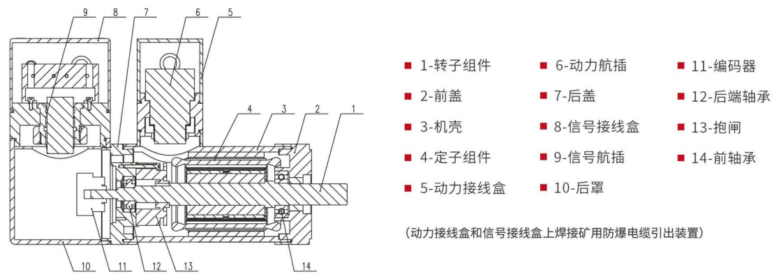
惠斯通矿用防爆电机的结构：
