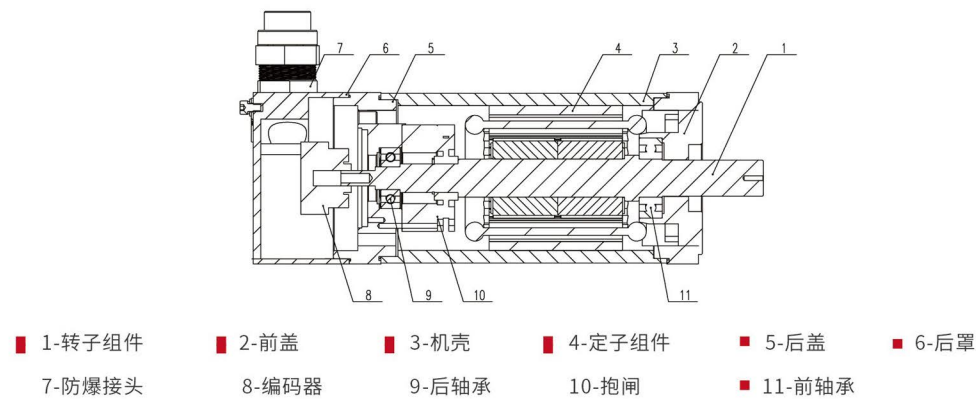
惠斯通隔爆型伺服电机的结构：
